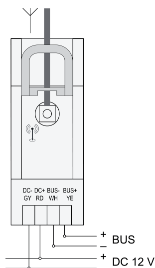
Afbeelding 2: Aansluitschema
