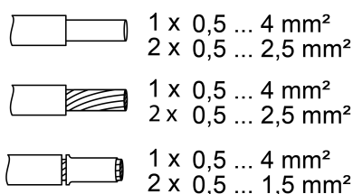
Bilde 4: Klembart ledertverrsnitt
