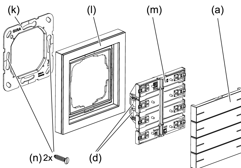
рисунок 5: Монтаж устройства
