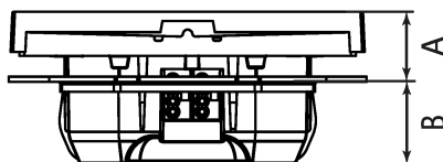
рисунок 11: Монтажные размеры
