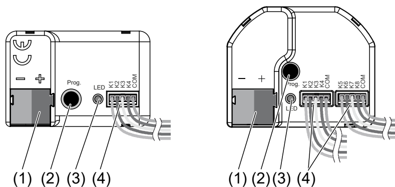
Bild 1: Geräteaufbau
