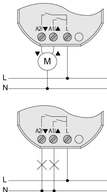
рисунок 5: Подключение нагрузки
