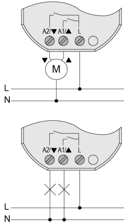
рисунок 5: Подключение нагрузки
