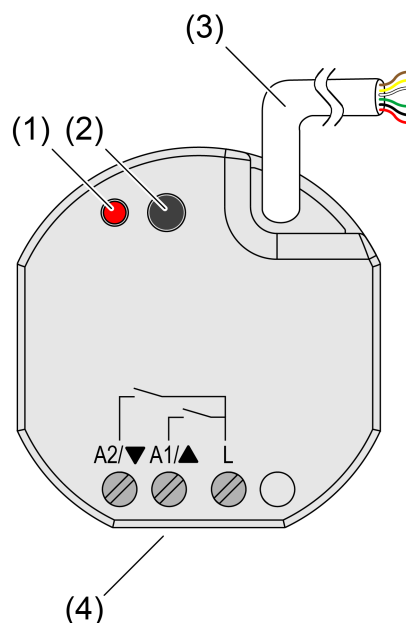
рисунок 1: Конструкция прибора
