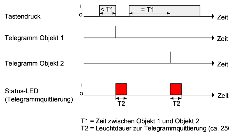
Bild 26: Beispiel zum Bedienkonzept "Kanal 1 oder Kanal 2"
