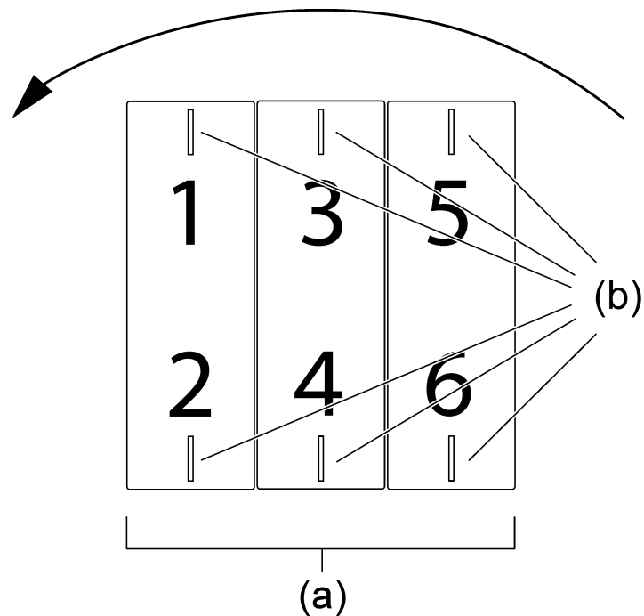
Bild 2: Geräteaufbau 3fach (Einbaulage "Um -90° gedreht", senkrechte Bedienwippen)
