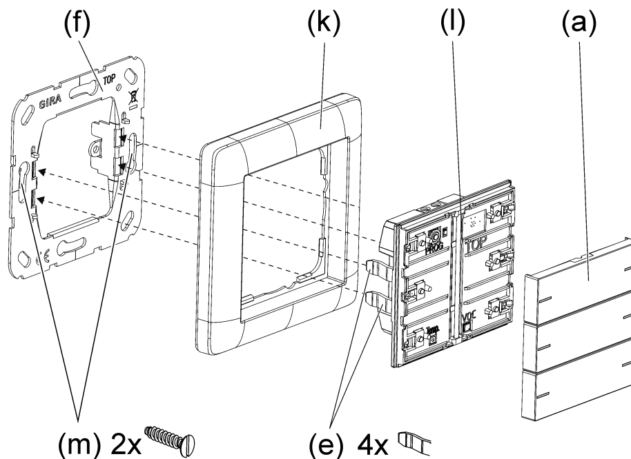
Bild 6: Gerät montieren
