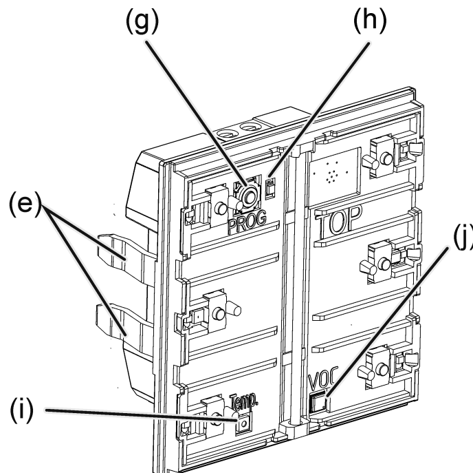
Bild 5: Tastsensor
