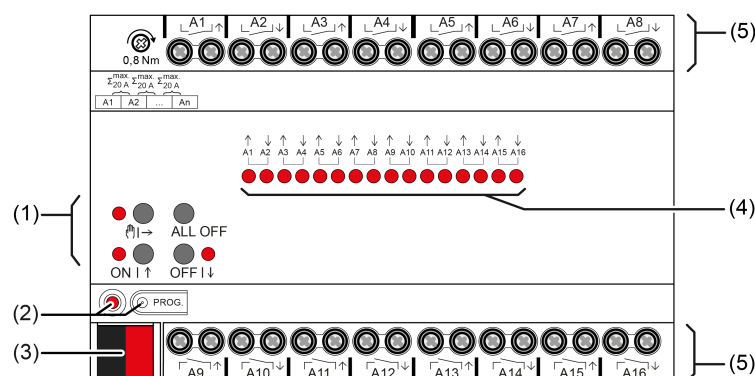
图像 1: 设备结构
