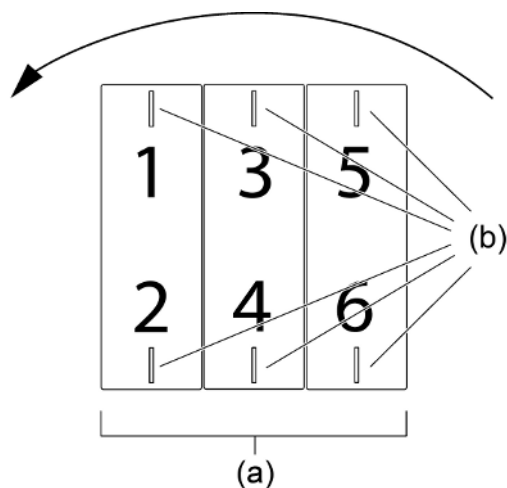
Figura 2: Estructura del aparato triple (posición de montaje "girado en -90^\circ ", interruptores basculantes de mando verticales)
