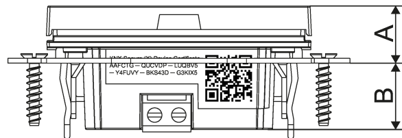
Afbeelding 11: Inbouwmaten
