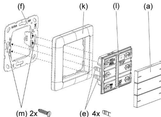
Afbeelding 5: Apparaat monteren
