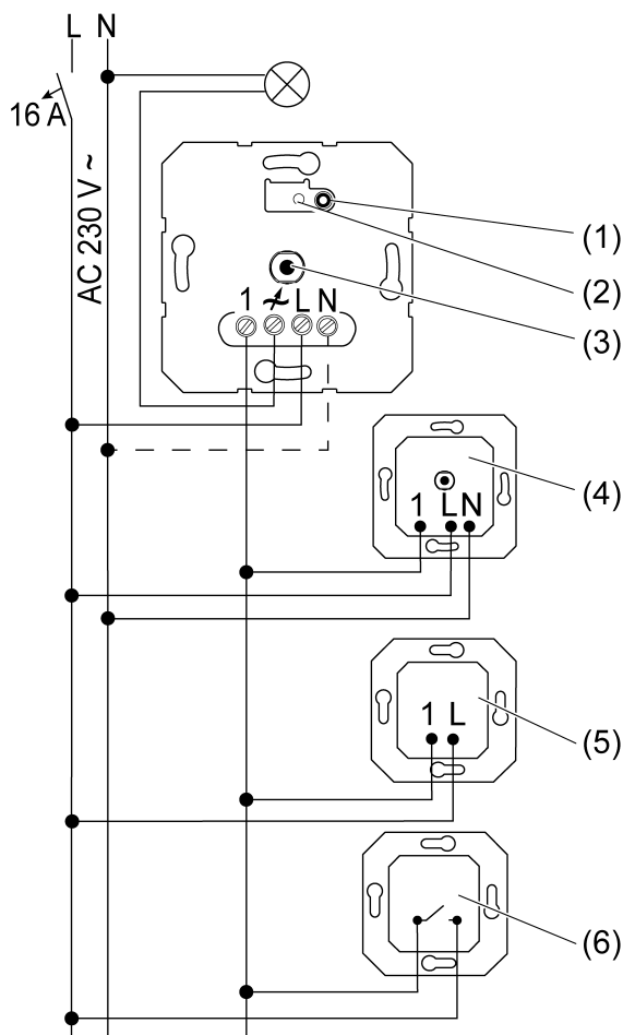
Kuva 3: Liitântäkaavio valinnaisilla alaliittymillä
