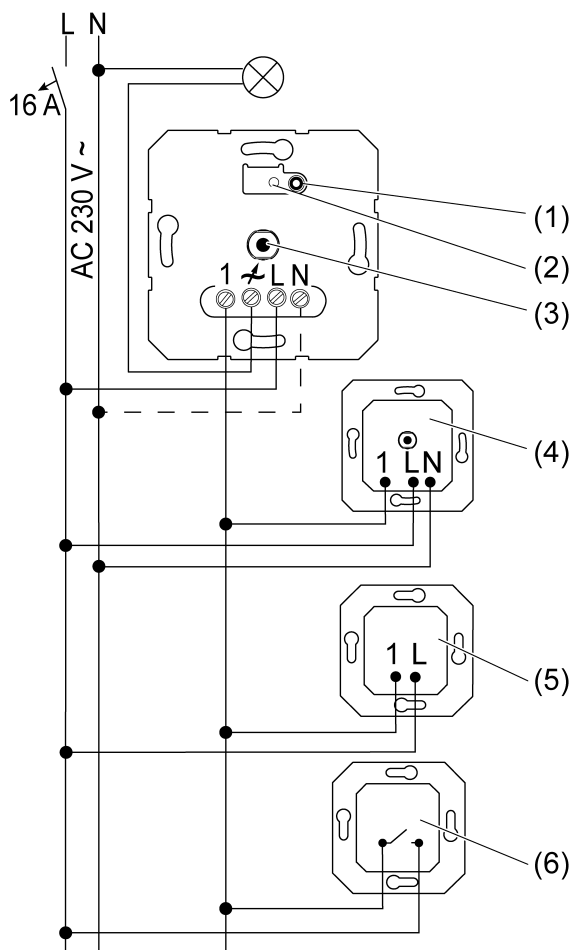
Imagem 3: Esquema de ligações com ramais opcionais
