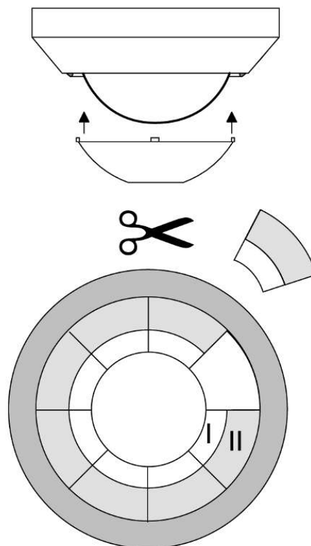
Bild 11: Aufsteckblende
