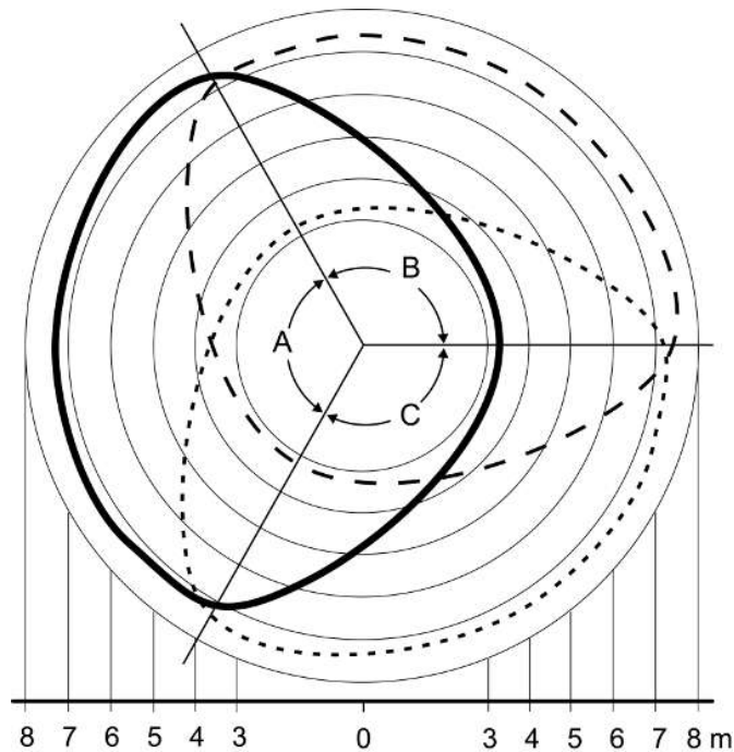
Bild 5: Erfassungsfeld Bereich A, B und C, Montagehöhe 2,50 m
