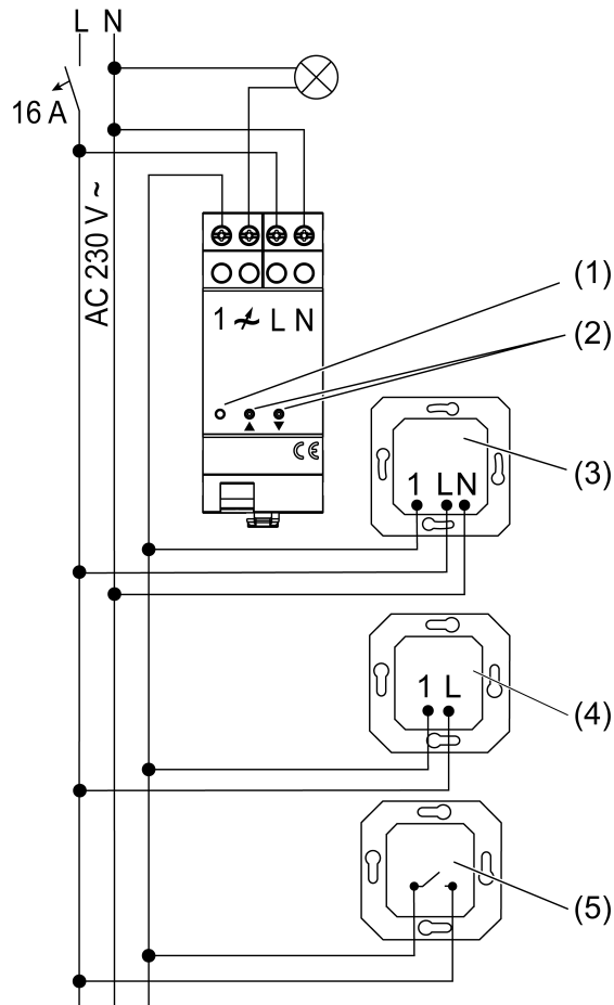
Kuva 1: Liitântäkaavio
