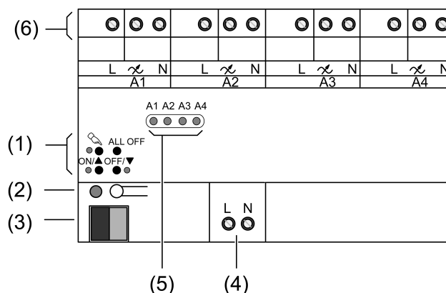
Figura 2: Vista attuatore regolazione di luminosità quadruplo
