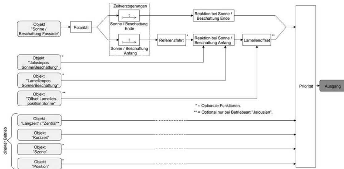
Bild 18: Funktionsschaltbild des einfachen Sonnenschutzes
