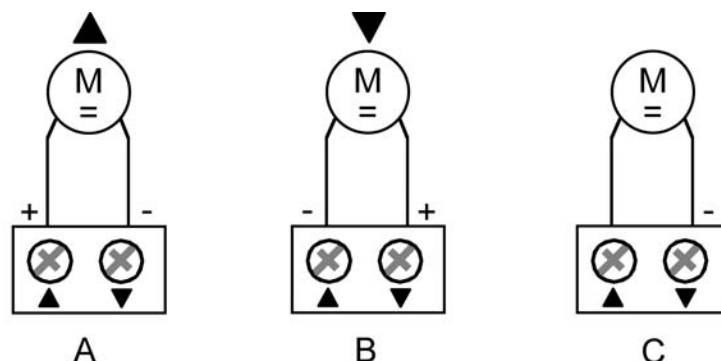
Bild 3: Polung an den Antriebsmotoren in Abhängigkeit der Fahrtrichtung (A und B) und bei gestopptem Antrieb (C).
