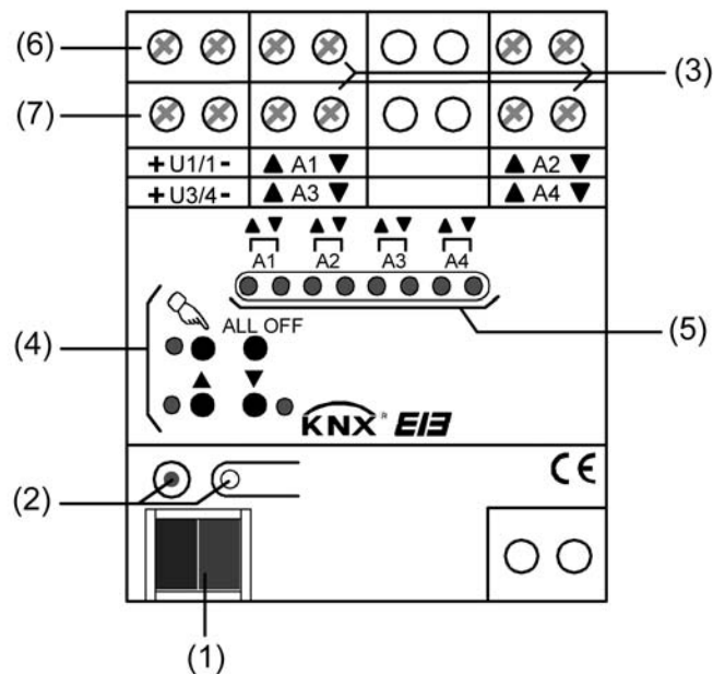
Bild 1: Geräteaufbau
