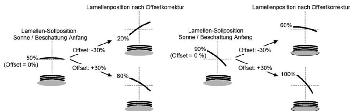
Bild 21: Funktionsweise des Lamellenoffsets als Beispiel (beispielhaft für Lamellentyp 1 / Lamellentyp 2 sinngemäß gleich)
