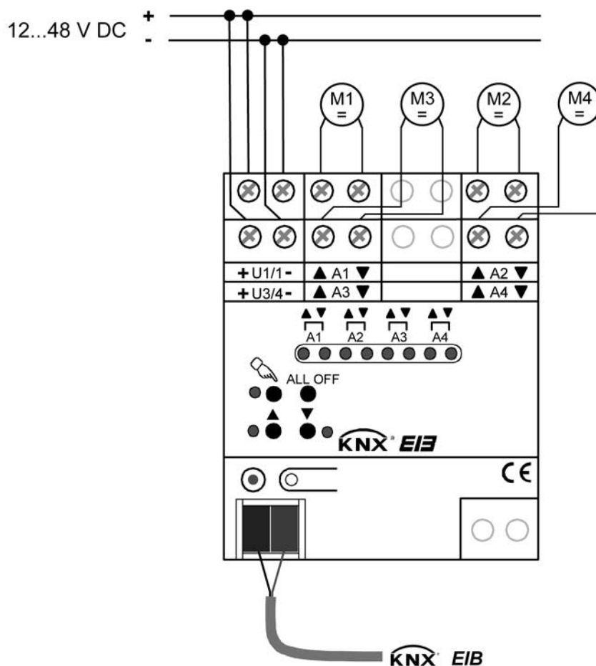
Bild 2: Elektrischer Anschluss
