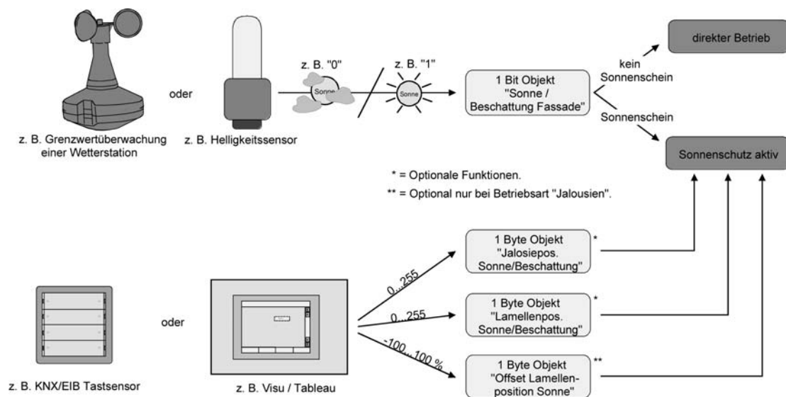
Bild 17: Prinzipschaltbild des einfachen Sonnenschutzes
