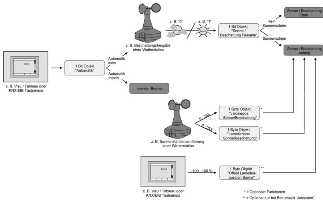
Bild 19: Prinzipschaltbild des erweiterten Sonnenschutzes (zur Vereinfachung ohne Sperrfunktionen)
