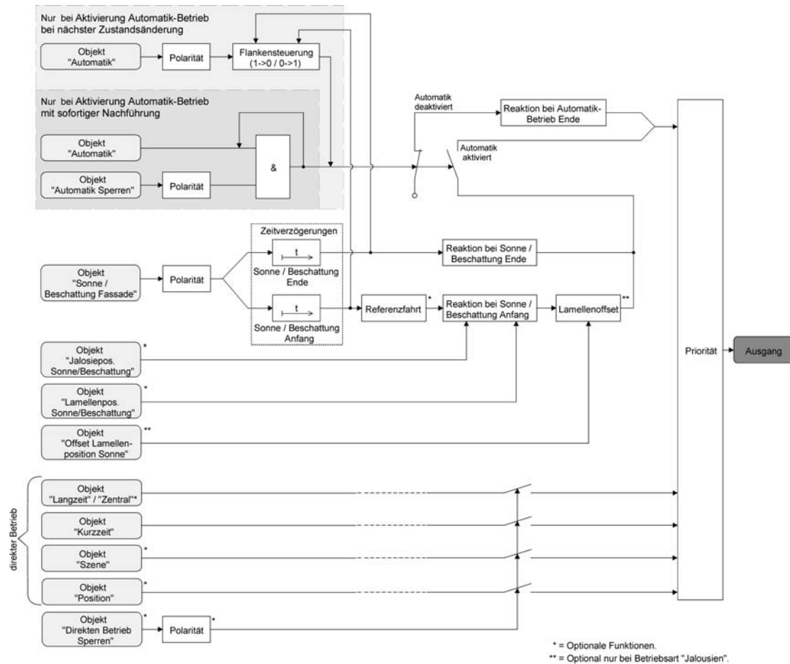
Bild 20: Funktionsschaltbild des erweiterten Sonnenschutzes
