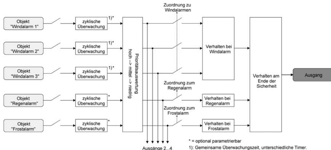
Bild 15: Funktionsschaltbild der kanalorientierten Sicherheitsfunktionen
