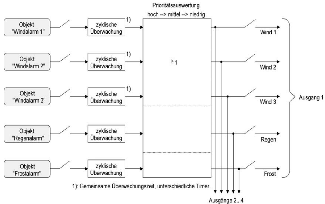
Bild 7: Funktionsschaltbild der Sicherheitsfunktionen
