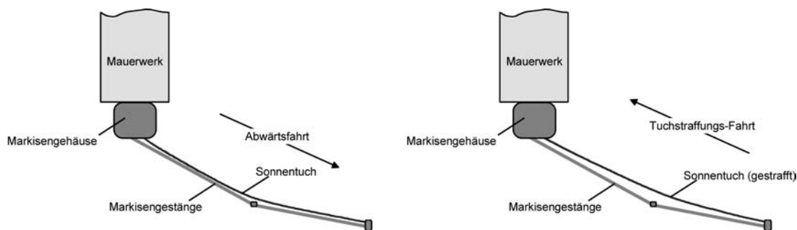
Bild 29: Tuchstraffung einer Markise
