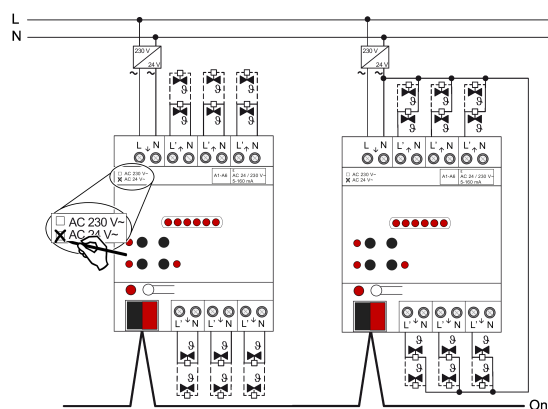
рисунок 4: Подключение для сервоприводов 24 В перем. тока
