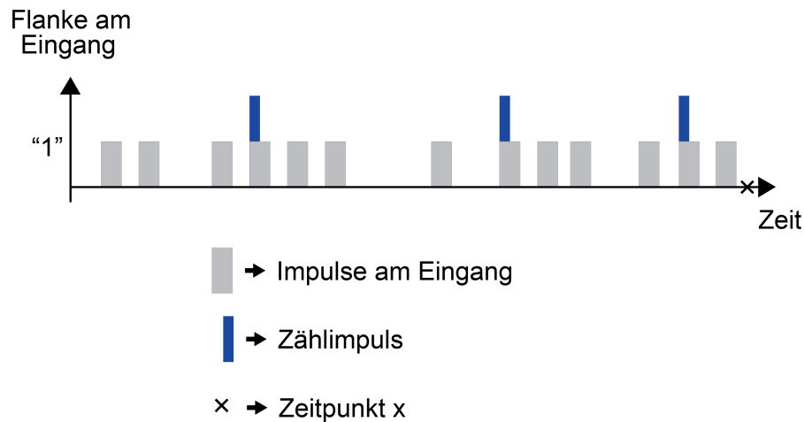
Bild 13: Beispiel zur Einstellung der Impulse am Eingang pro Zählimpuls
