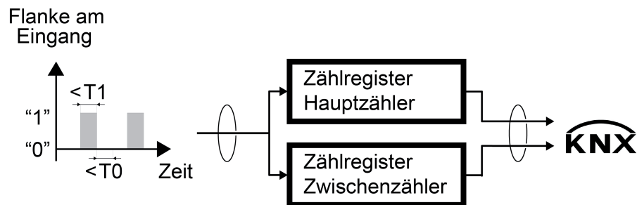
Bild 12: Funktionsschema des Impulszählers
