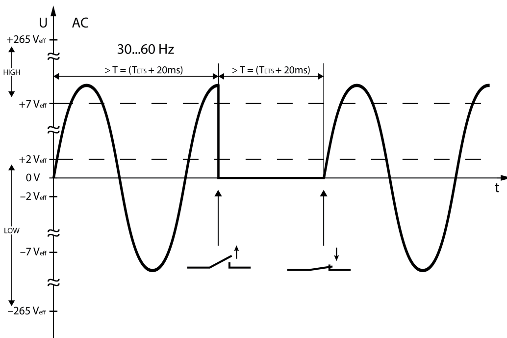
Bild 7: Beispiel eines Signalverlaufes eines Wechsellspannungssignals (AC)
