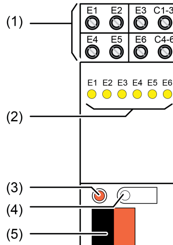
Bild 1: Geräteaufbau Binäreingang 6fach 10...230 V
