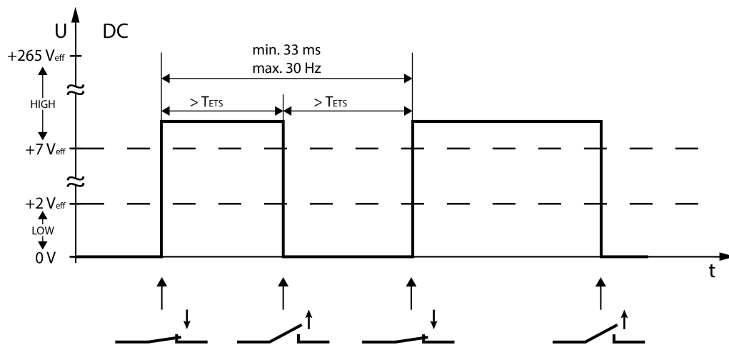
Bild 6: Beispiel eines Signalverlaufes eines Gleichspannungssignals (DC)
