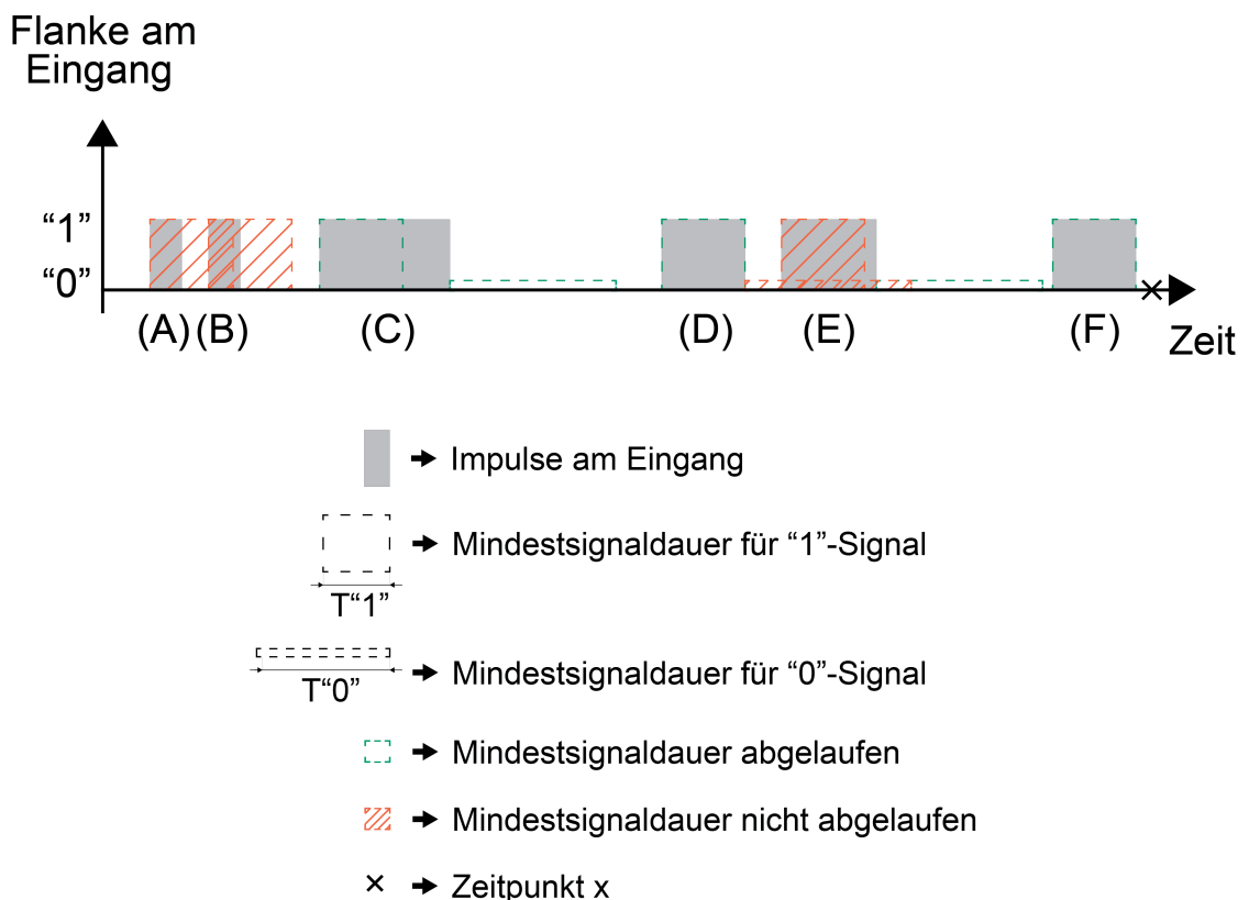
Bild 15: Beispiel zur Einstellung der Mindestsignaldauer
