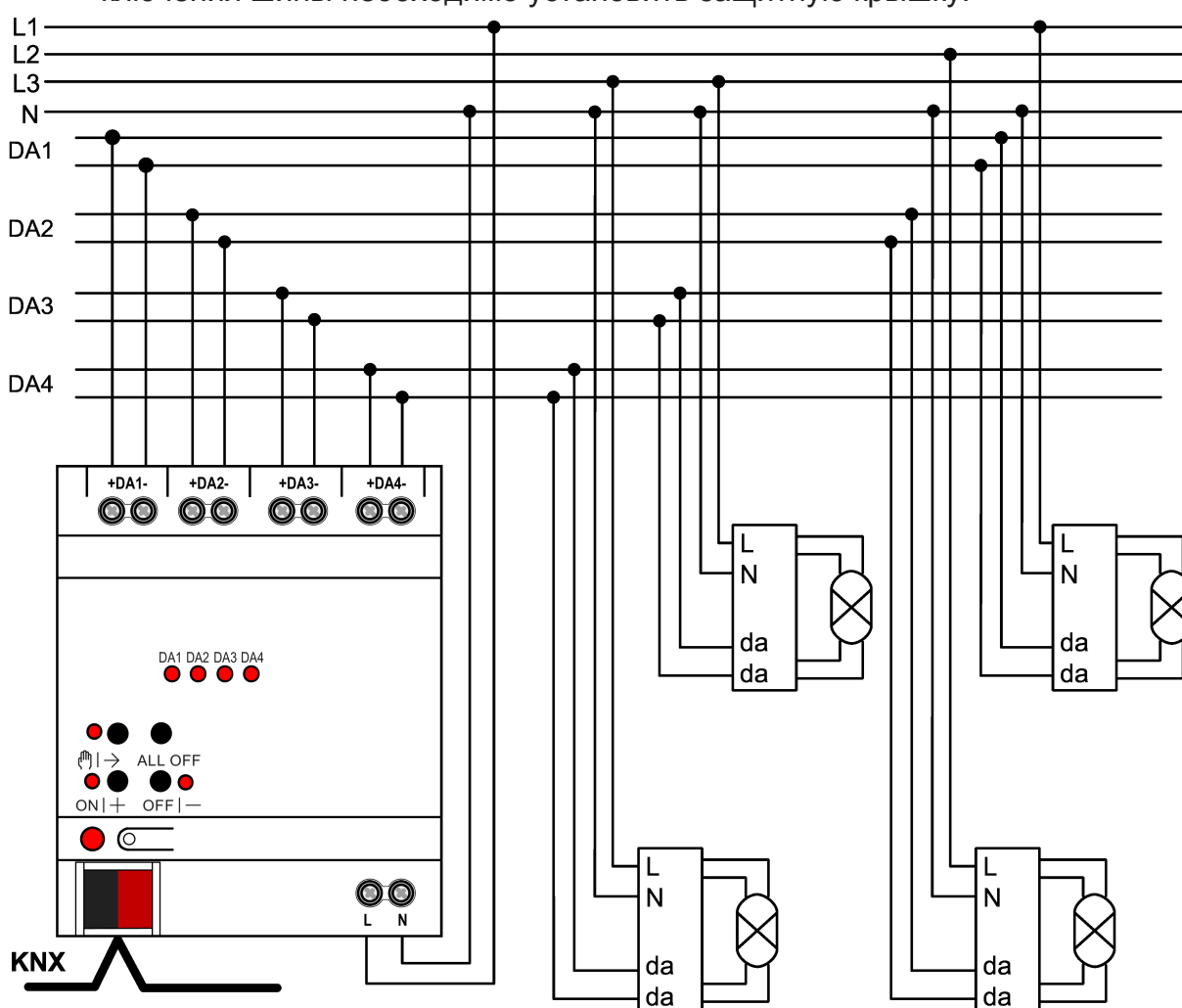
рисунок 2: Пример подключения
