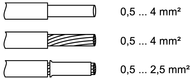
Figura 5: Secciones de cable conectables a borne
