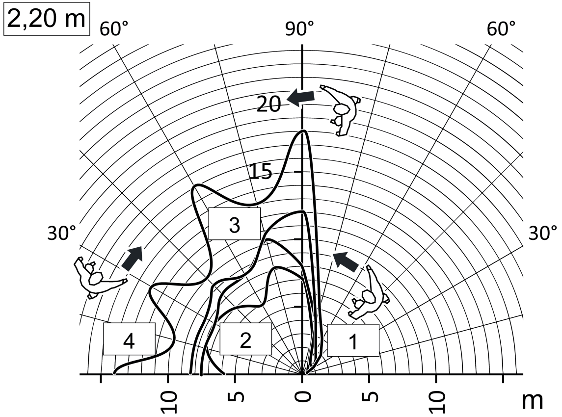
Bild 13: Reichweite bei tangentialer Bewegungsrichtung, Einbauhöhe 2,20 m, nur ein Sensor aktiv
