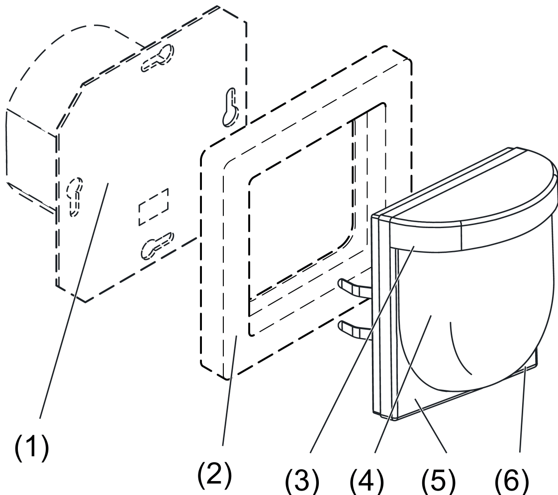
Bild 1: Geräteaufbau
