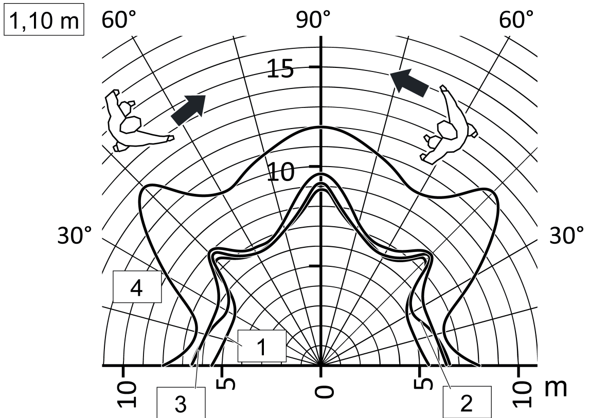
Bild 11: Reichweite bei tangentialer Bewegungsrichtung, Einbauhöhe 1,10 m
