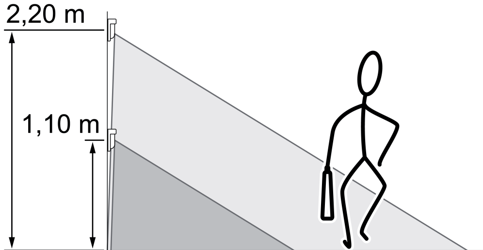
Bild 8: Erfassungsfeld und Einbauhöhe
