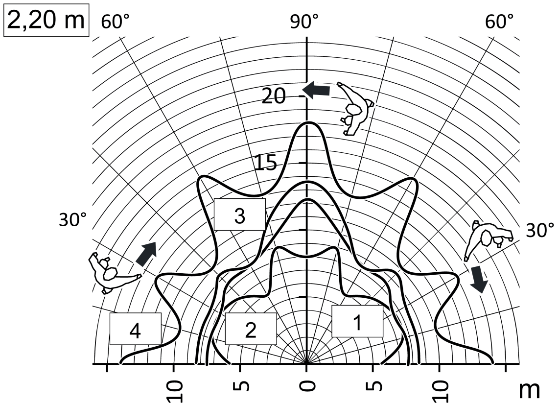
Bild 9: Reichweite bei tangentialer Bewegungsrichtung, Einbauhöhe 2,20 m
