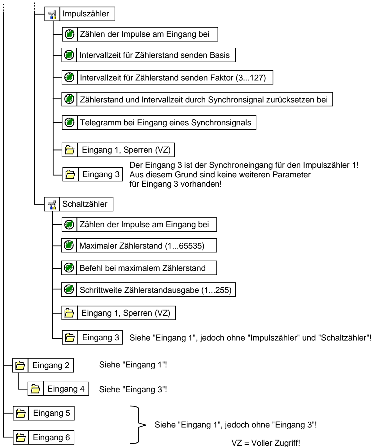
Parameterbild (Teil 5 von 5)
