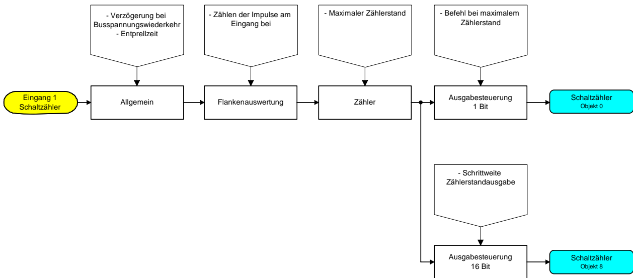
Funktionsschaltbild (z. B. Eingang 1 Funktion "Schaltzähler")
