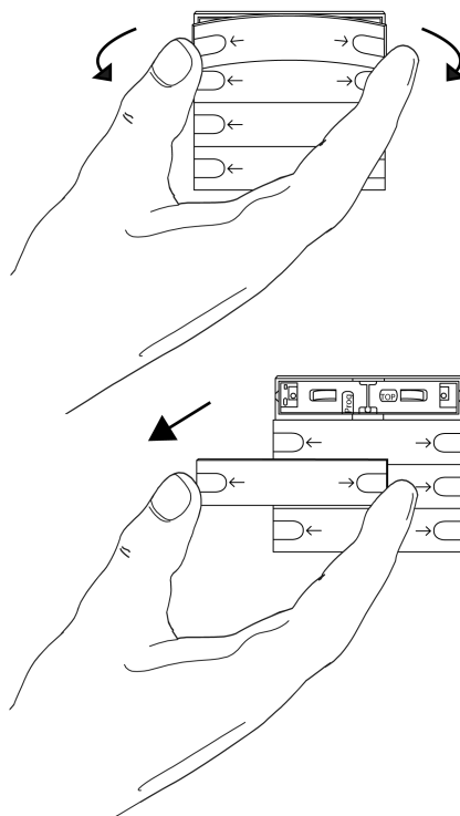
рисунок 5: Демонтаж клавиши для ввода в эксплуатацию
