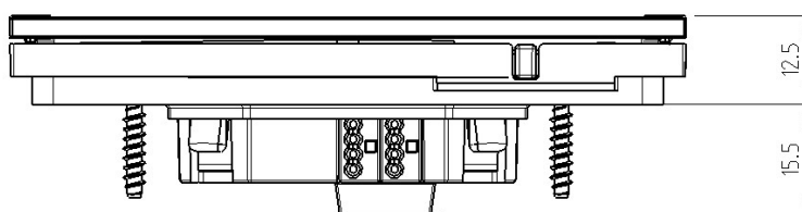
рисунок 7: Монтажные размеры
