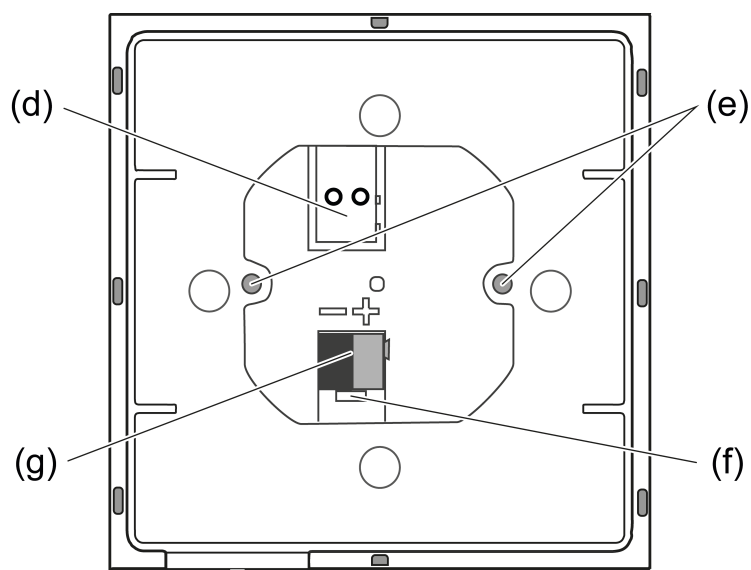
рисунок 2: Конструкция прибора – задняя сторона
