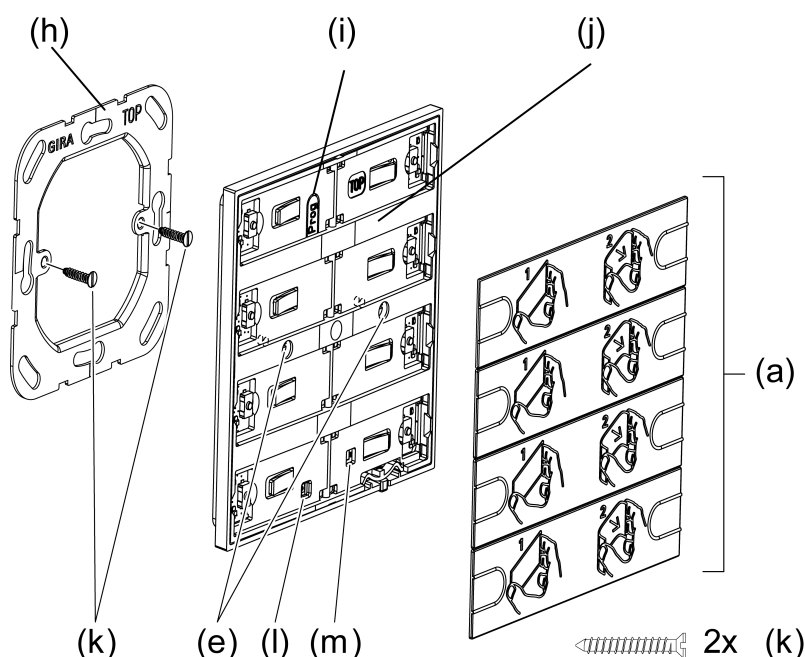
рисунок 3: Монтаж устройства
