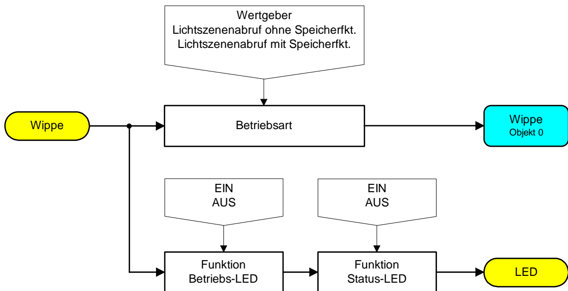
Funktionsschaltbild
