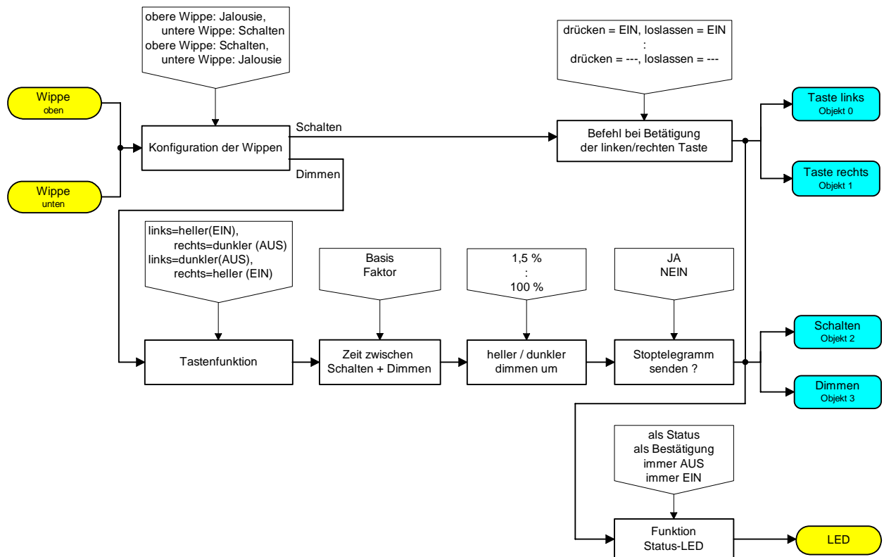
Funktionsschaltbild
