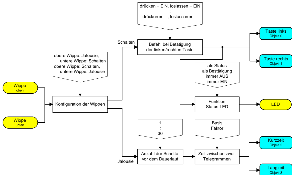
Funktionsschaltbild
