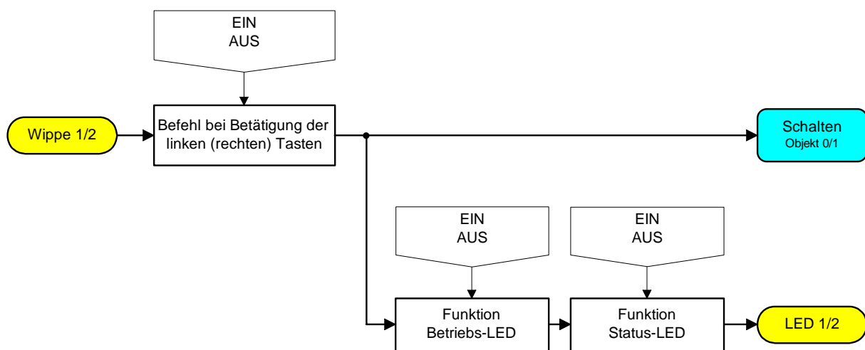
Funktionsschaltbild
