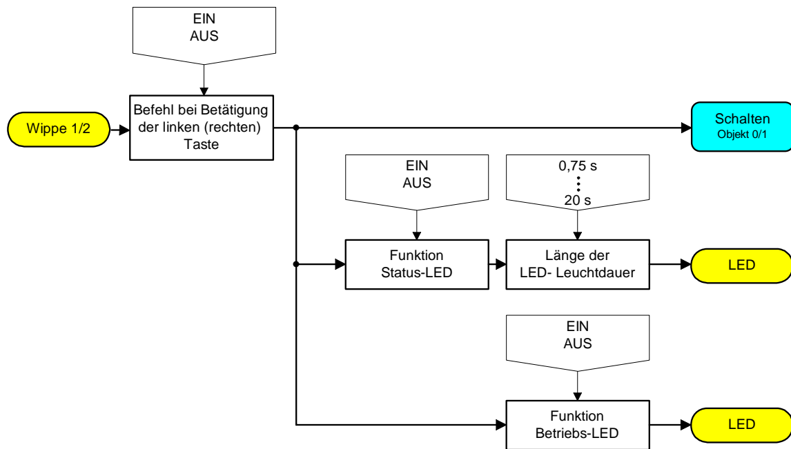
Funktionsschaltbild
