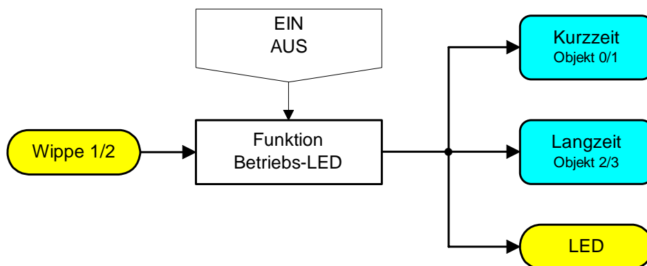
Funktionsschaltbild
