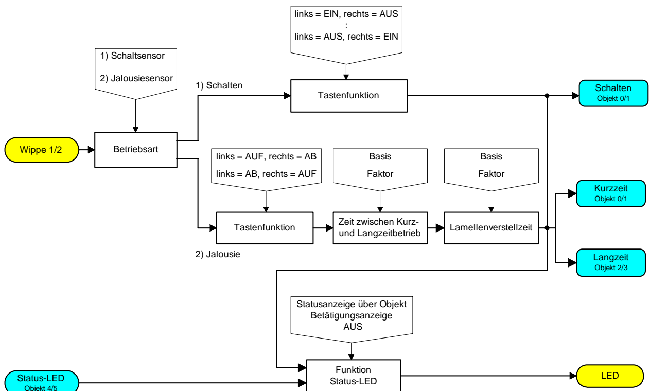
Funktionsschaltbild
