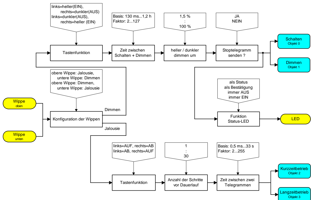
Funktionsschaltbild
